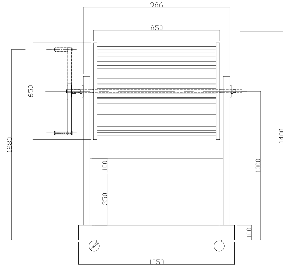
正面図
